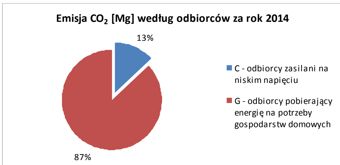
Wykres 15 . Emisja CO 2 [Mg] według odbiorców energii za rok 2014 (źródło: opracowanie własne)
