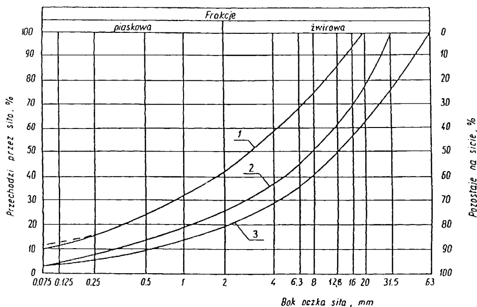
1-3 kruszywo na podbudowę pomocniczą (dolną warstwę)
